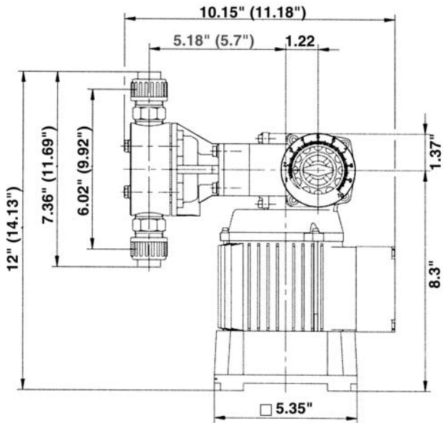
MEMDOS MD E24 and (E120) Dimensions
